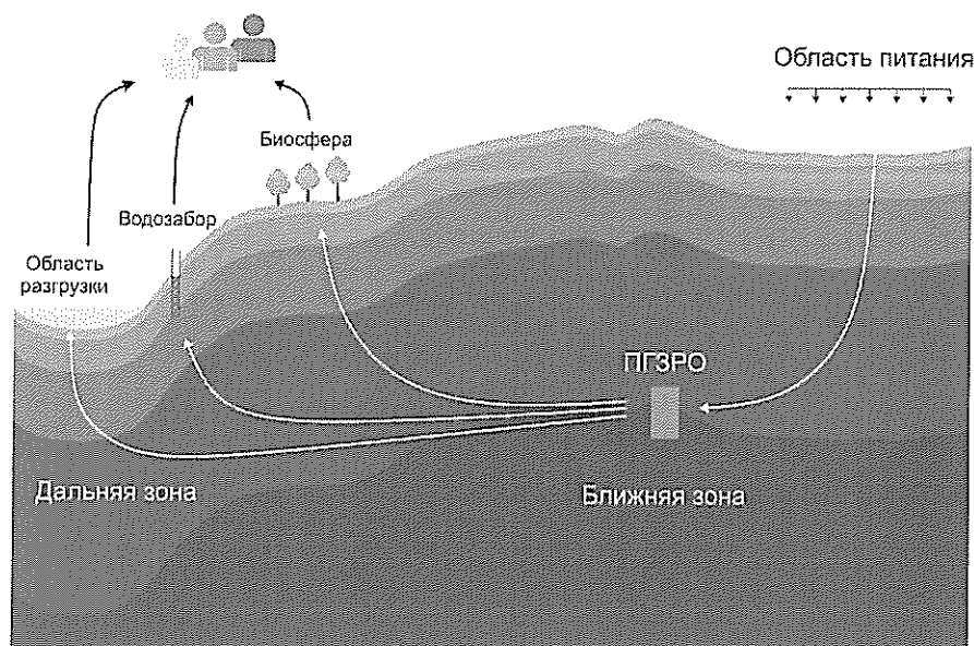
Рис. 1. Концептуальная модель системы захоронения РАО
